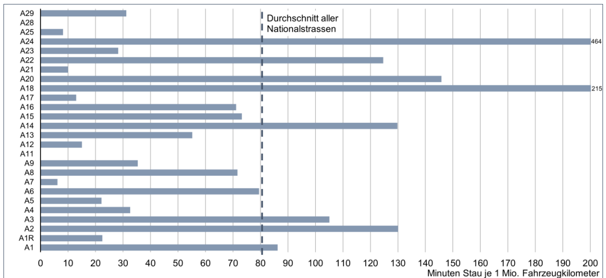
Abbildung 27: Fahrleistungsbezogene Stauintensität 2022 nach Nationalstrassen (inkl. NEB-Strecken)
