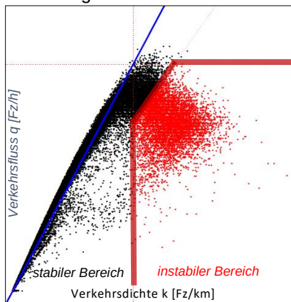
Abbildung 59 Fundamentaldiagramm für eine Zählstelle in eine Fahrrichtung
