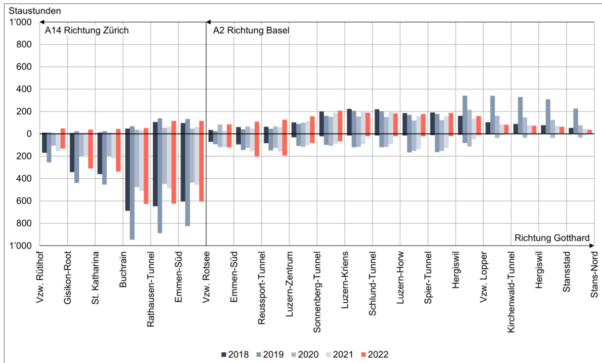
Abbildung 36: Entwicklung der Stautunden auf A14 und A2 zwischen Rütihof und Stans Quellen: ASTRA: VMON, Viasuisse
