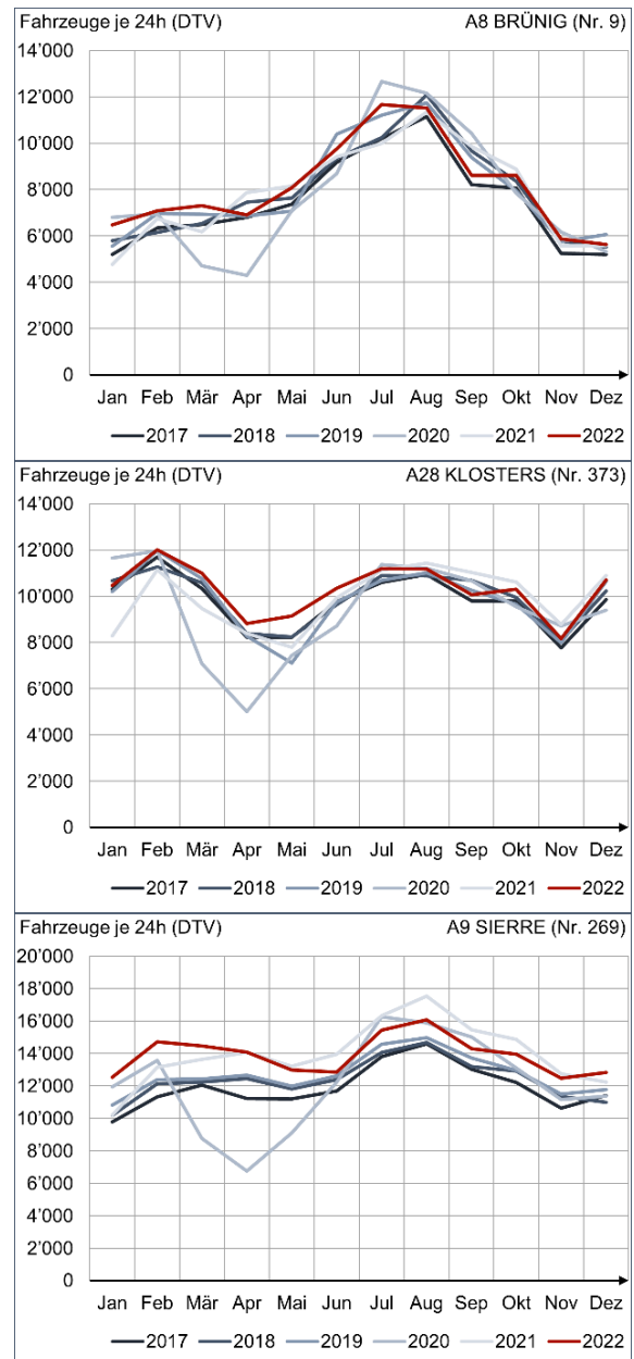
Abbildung 18: Ausgewählte Jahresganglinien DTV im Corona-Jahr 2020 für das Jahr 2022
