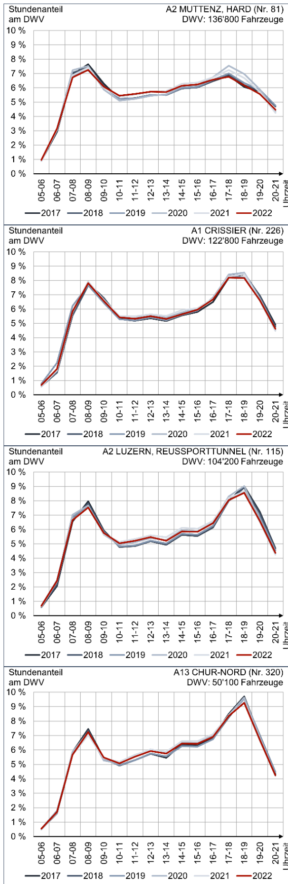
Abbildung 20: Tagesganglinien DWV an ausgewählten Zählstellen aus allen Landesteilen Quellen: ASTRA: SASVZ, ASTRA: VMON
