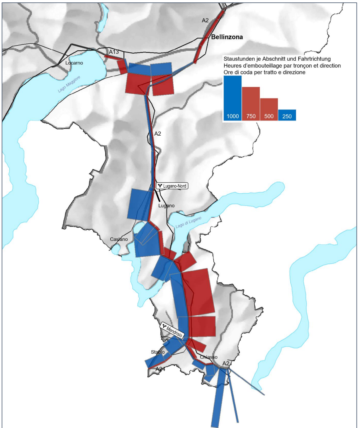
Abbildung 44: Staustunden 2022 auf den Nationalstrassen im Tessin Quellen: ASTRA: VMON, Viasuisse
